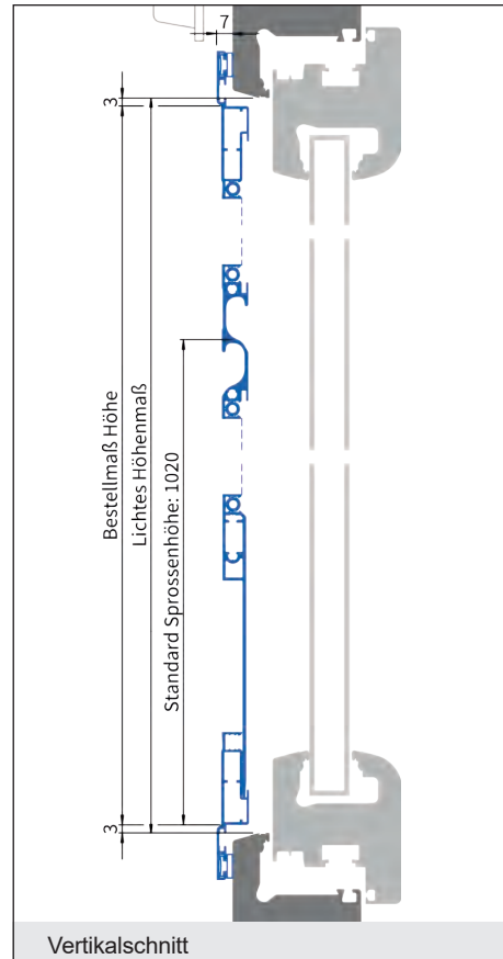
Vertikalschnitt
