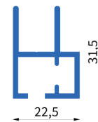
Art. Nr.: 1101 Bez.: Führungsschiene für 2-schienige Schiebeanlagen
