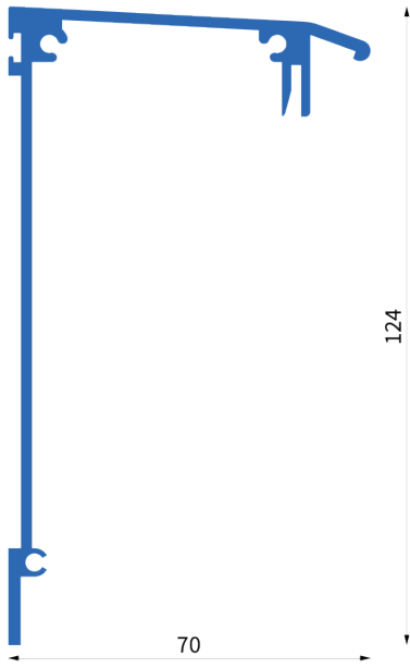
Art. Nr.: 1736 Bez.: Lüftungsprofil
