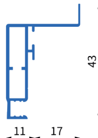
Art. Nr.: 1204 Bez.: Spannrahmenprofil SEC mit Fahne 27 mm
