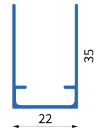
Art. Nr.: 2550 Bez.: Obere Führungsschiene
