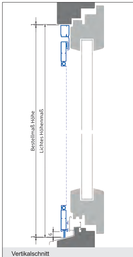
Vertikalschnitt
