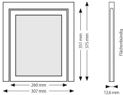
Haustierklappe groß Art.-Nr. 5505
