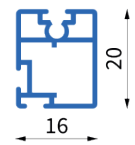
Art. Nr.: 2309 Bez.: Verbindungsprofil
