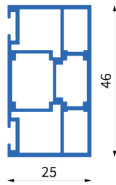
Art. Nr.: 1041 Bez.: Einbaurahmenprofil verstärkt für Drehtüren
