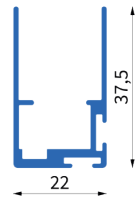
Art. Nr.: 2556 Bez.: Kombi-Rahmenprofil mit Bürstenführung
