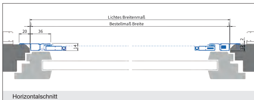
Horizontalschnitt
