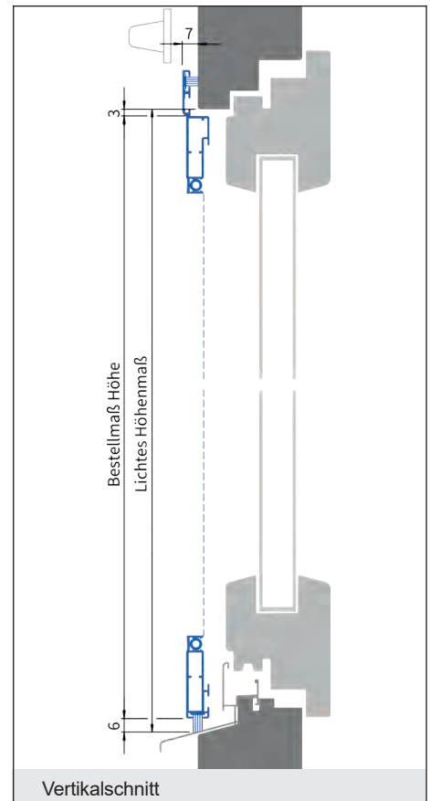
Vertikalschnitt
