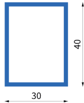
Art. Nr.: 1012 Bez.: Vierkantprofil 30 x 40 x 2 mm
