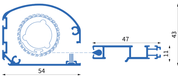
Art. Nr.: 2330 Gewebegröße 160 cm, grau Art. Nr.: 2335 Gewebegröße 160 cm, schwarz Art. Nr.: 2340 Gewebegröße 240 cm, grau Art. Nr.: 2345 Gewebegröße 240 cm, schwarz Bez.: Rollokassette mit Zugschiene
