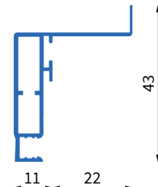
Art. Nr.: 1206 Bez.: Spannrahmenprofil SEC mit Fahne 32 mm
