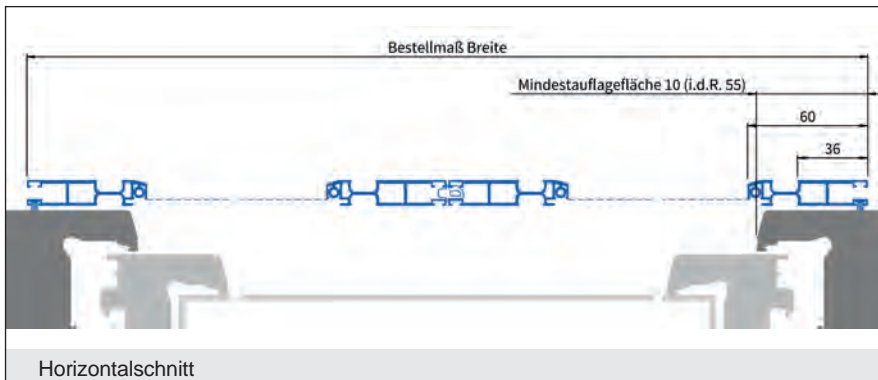
Horizontalschnitt
