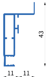
Art. Nr.: 1202 Bez.: Spannrahmenprofil SEC mit Fahne 21 mm
