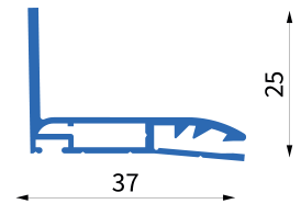
Art. Nr.: 1709 Bez.: Lichtschachtprofil, abgerundet mit Fahne
