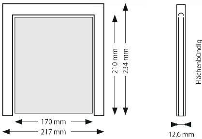
Haustierklappe klein Art.-Nr. 5504
