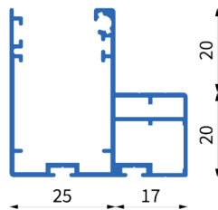
Art. Nr.: 2307 Bez.: Rollo Führungsschiene, breit
