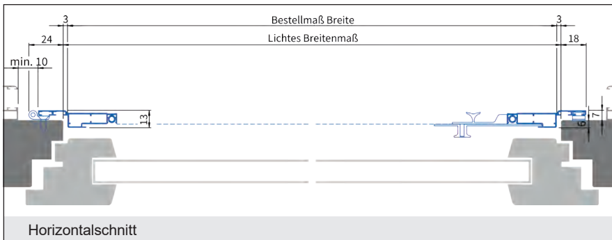
Horizontalschnitt
