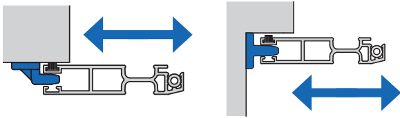
Frontale Befestigung
