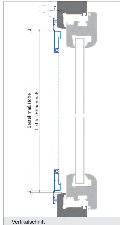
Vertikalschnitt
