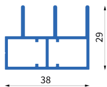
Art. Nr.: 1106 Bez.: Führungsschiene für 3-schienige Schiebeanlagen
