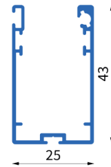
Art. Nr.: 2308 Bez.: Rollo Führungsschiene mit Befestigungsnut
