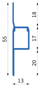
Art. Nr.: 1326 Bez.: Einbaurahmenprofil mit doppeltem Falz, gleichseitig
