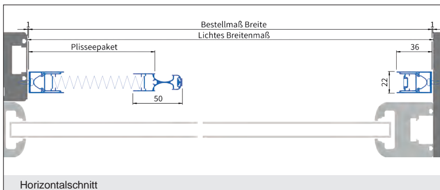
Horizontalschnitt
