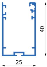
Art. Nr.: 2305 Bez.: Rollo Führungsschiene, schmal
