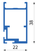
Art. Nr.: 2571 Bez.: Kombi-Rahmenprofil Laufschiene mit Bürstenführung
